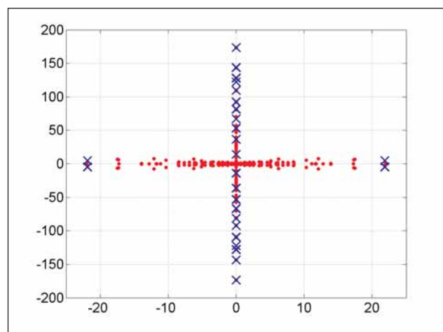
Bild 1: Eigenwertapproximationen
